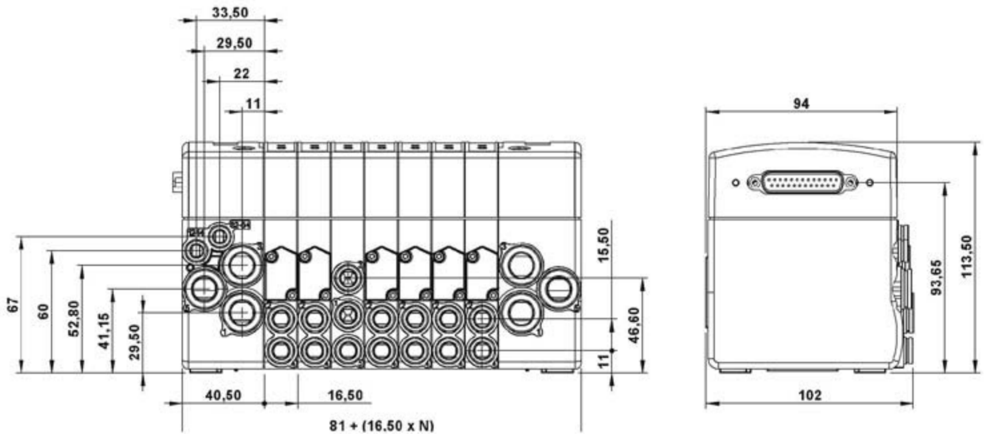
Dimensioni Kit Assemblaggio Assembling kit dimensions
