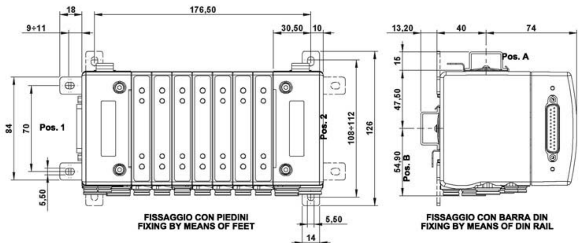
Dimensioni Kit Assemblaggio Assembling kit dimensions
