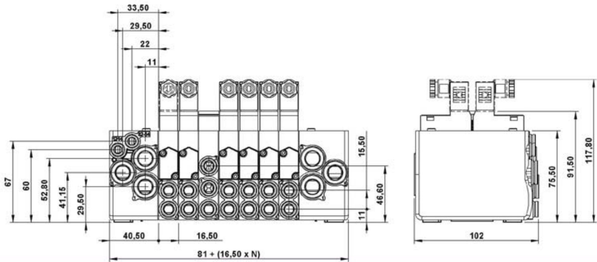
Dimensioni cablaggio multipolare Multipole cabling dimensions
